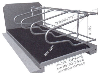
12. att. Kubisko guļvietu izmēri
