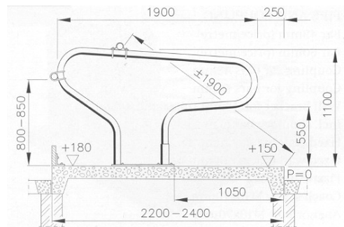
9. att. Sērņveida gulvietu izmēri
