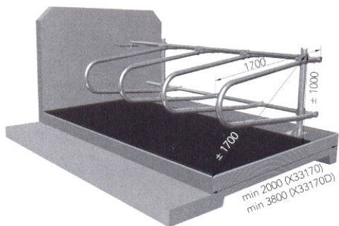
6. att. Gulvietas telītēm vecumā no 10 līdz 16 mēnešiem, kuras tur brīvājās turēšanas sistēmās
