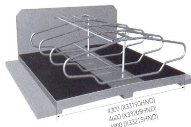
13. att. Kubiskās guļvietas
