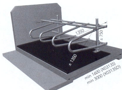
4. att. Gulvietas jaundzīvniekiem, kurus no 1–5 mēnešu vecumam tur brīvājās turēšanas sistēmās
