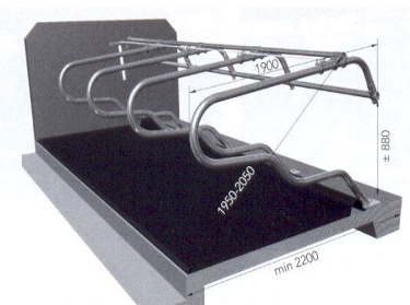
14. att. Kubisko guļvietu izmēri
