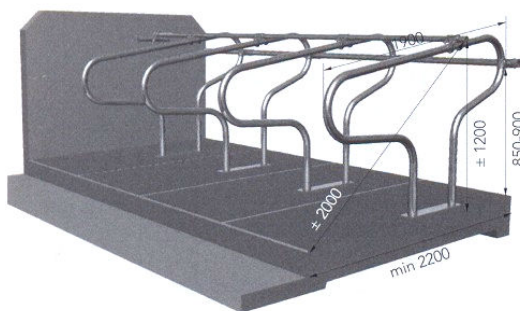
8. att. Mikstās sērņveida gulvietas
