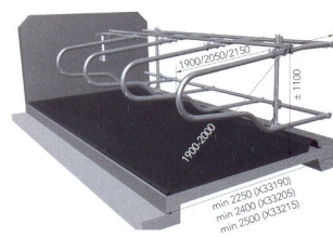
11. att. Kubisko guļvietu izmēri
