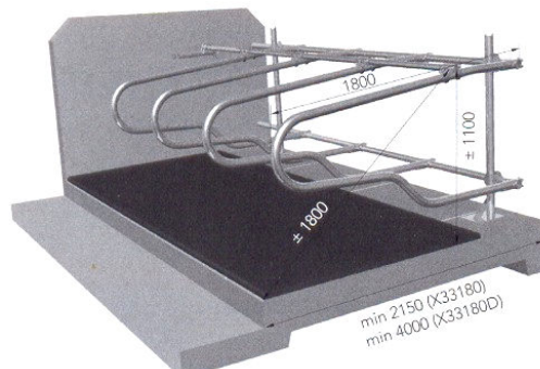
7. att. Gulvietas telītēm vecumā no 16 līdz 22 mēnešiem, kuras tur brīvājās turēšanas sistēmās
