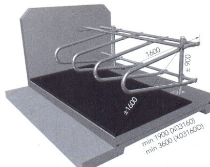
5. att. Gulvietas jaundzīvniekiem, kurus no 5–12 mēnešu vecumam tur brīvājās turēšanas sistēmās
